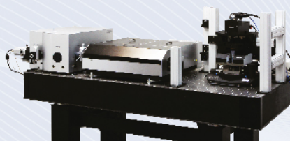
Sistema automatizado AFM-Raman, SNOM e TERS
