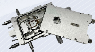
Platina de microtermometria para microscopia ótica e espectrometria
