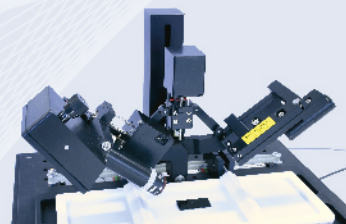
Microscópio de ângulo de Brewster
