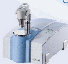
FTIR
