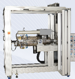
Célula PVT 400/1000 visibilidade total PVT FV2
